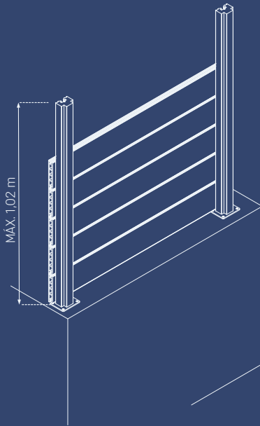
FIXAÇÃO COM FIXADORES EM BASE DE BETÃO FIJACIÓN CON FIJADORES EN BASE DE HORMIGÓN
