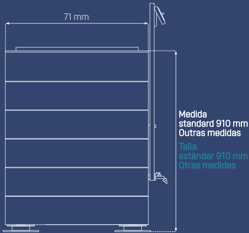
Alçado lateral Alzado lateral
