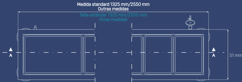
Planta Plano de planta
