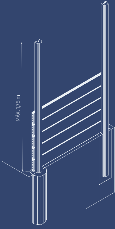
FIXAÇÃO DIRETA NO SOLO COM MACIÇO DE BETÃO FIJACIÓN DIRECTA EN EL SUELO COM MACIZADO DE HORMIGÓN
