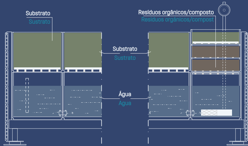
Corte BB Corte BB
