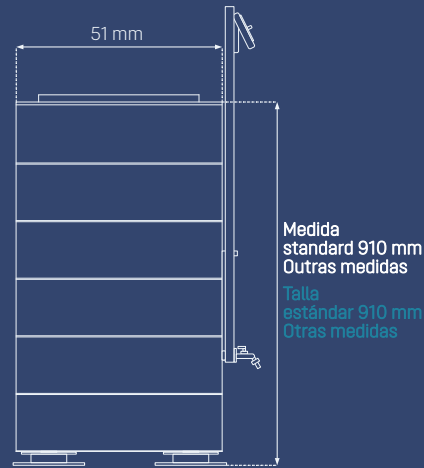
Alçado lateral Alzado lateral
