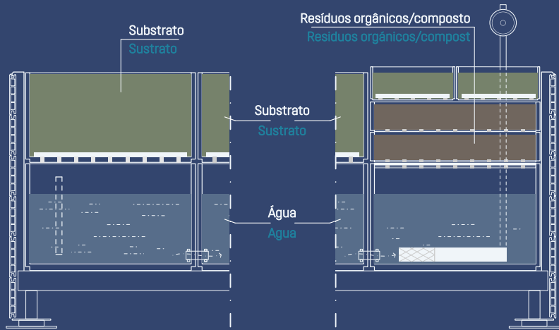
Corte AA Corte AA
